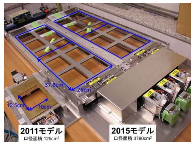
図3: 多段シフター1号機(左)と2号機(右)
