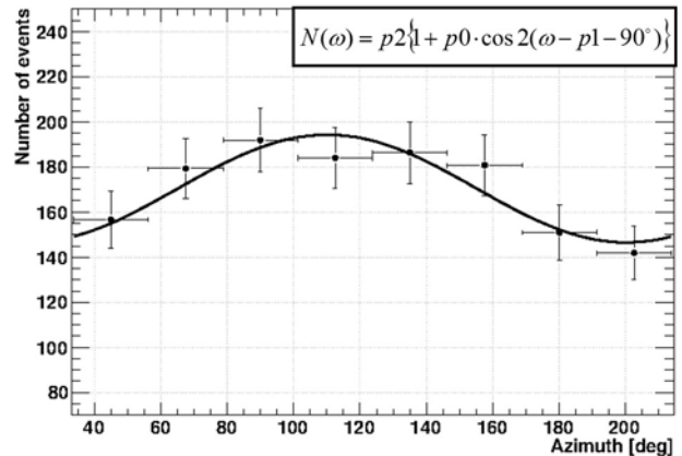
図2: 直線偏光ガンマ線による電子対の方位角分布
