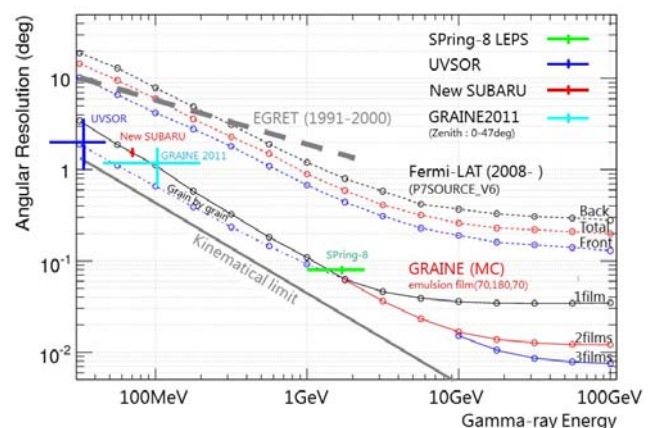
図1: ガンマ線に対する角度分解能(Fermi 望遠鏡、原子核乾板のシミュレーションと実験データ)
