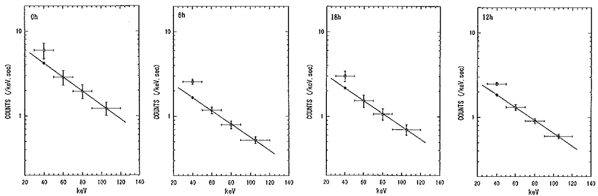
図7 各MLTにおけるエネルギースペクトル。直線はE2～E4でbest fitさせて求めたもの。菱形はfitさせたパラメーターを用いて推定した E_1 ( E_{1\text{ est}} )。
