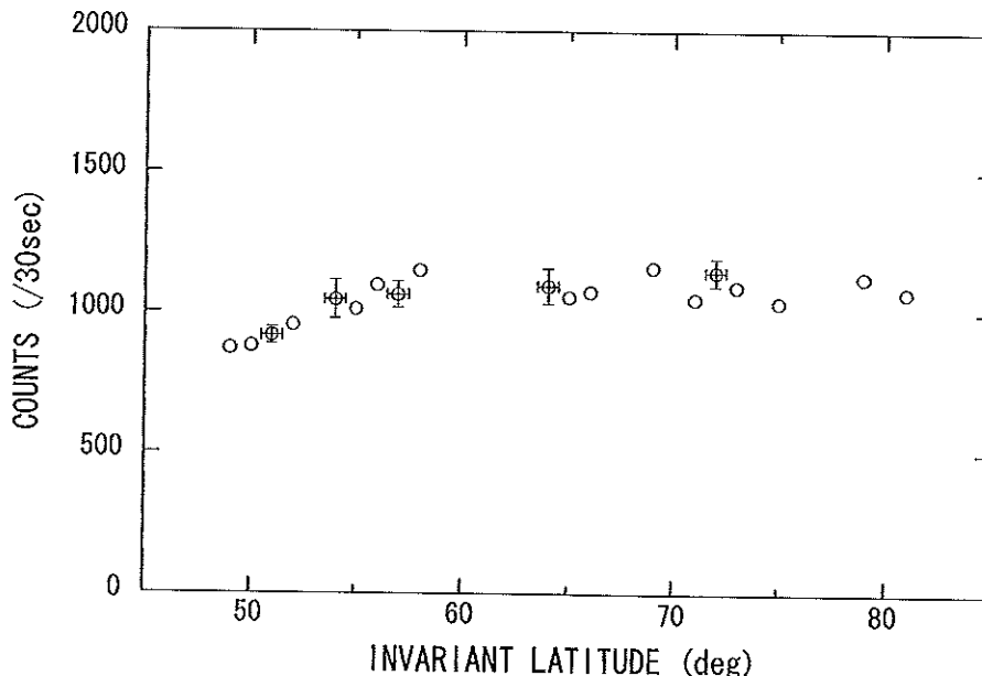
図2 大気硬X線バックグラウンド強度の不変磁気緯度に対する変化
