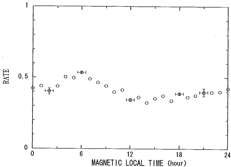
図8 E1_{est} に対する (E1_{obs} - E1_{est}) の割合
