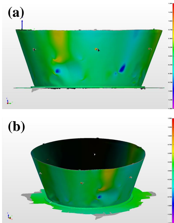
Fig.6 ノズル展開試験前後形状変化 カラーマップ (a)水平方向 (b)俯瞰図
