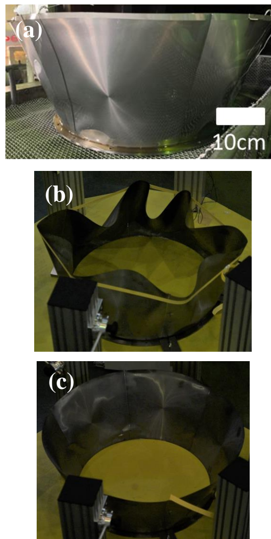
Fig.5 実物大超弾性ロケットノズル模型 (a)展開前 (b)折畳中 (c)展開後
