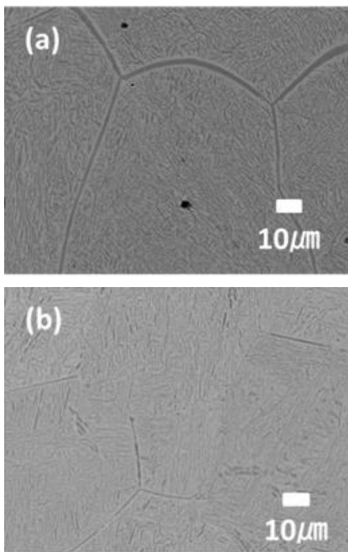
Fig.4 (a)溶接+800°C10分焼鈍材 (b)溶接+850°C10分+875°C10分溶体化 +825°C焼鈍+125°C1h時効材 SEM写真
