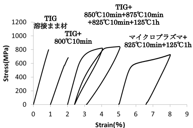
Fig.3 溶接部熱処理材の超弾性の変化
