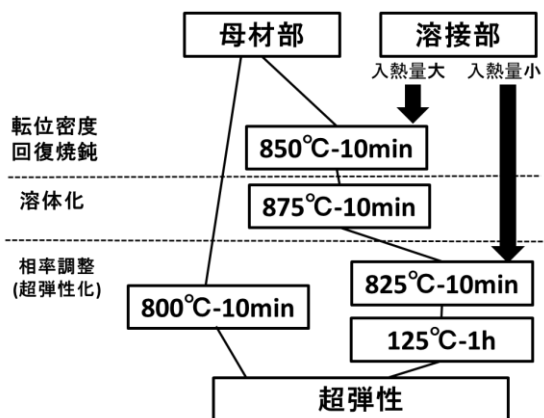
Fig.1 母材部・溶接部熱処理フローチャート
