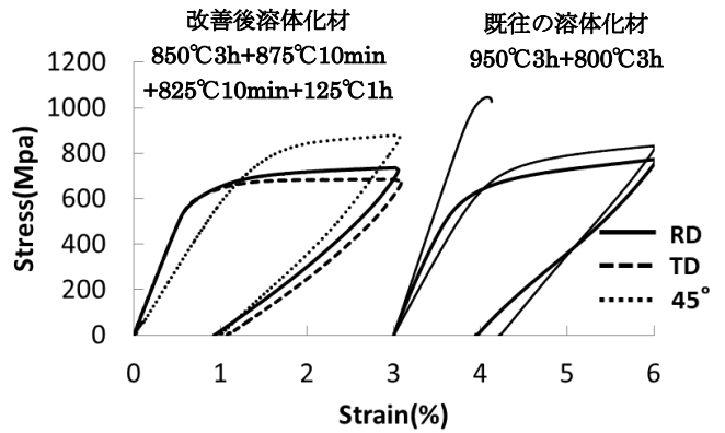
Fig.2 溶体化材母材部の超弾性の変化
