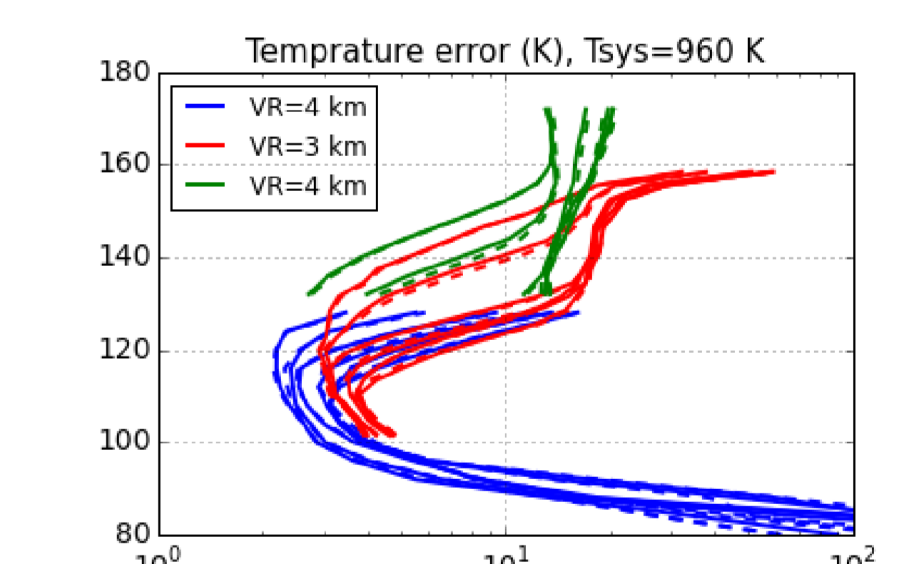
図5(右下): 2.06THz帯を利用して温度を観測する例。
