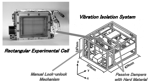
Fig.2 The apparatus for IML-2(1994).
