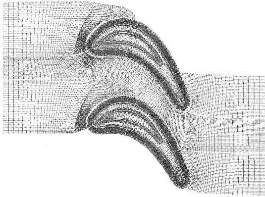
図 8: 熱伝導との連成用計算格子
