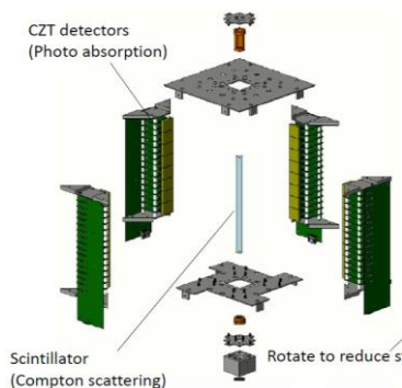
図 3 : X(L)-Calibur 偏光計の解体図。上方から入射した硬 X 線は、中心の散乱体で散乱され、周囲 4 辺を囲う CZT 半導体検出器で検出される。これにより散乱角が測定でき、その垂直方向が入射光子の偏光方向であると分かる。散乱体は、パッシブなベリリウム単体である。次回以降フライトでは、CZT 検出器の厚みを 2 mm から 0.8 mm に薄くし、バックグラウンドを低減させる。
